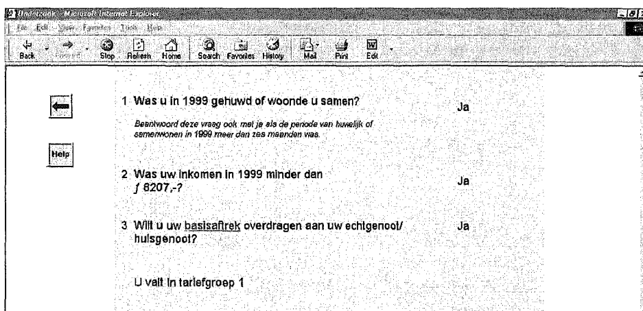
Afb. 2 Vraag-antwoordstructuur – Voorbeeldroute
